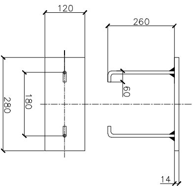
预埋件 M1
